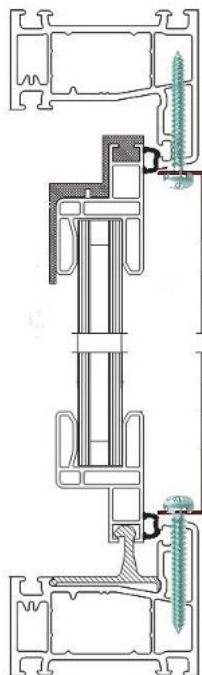
Ansicht von innen (Die Schrauben sind nur schematisch dargestellt und nicht sichtbar!)
